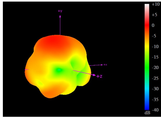
960MHz
