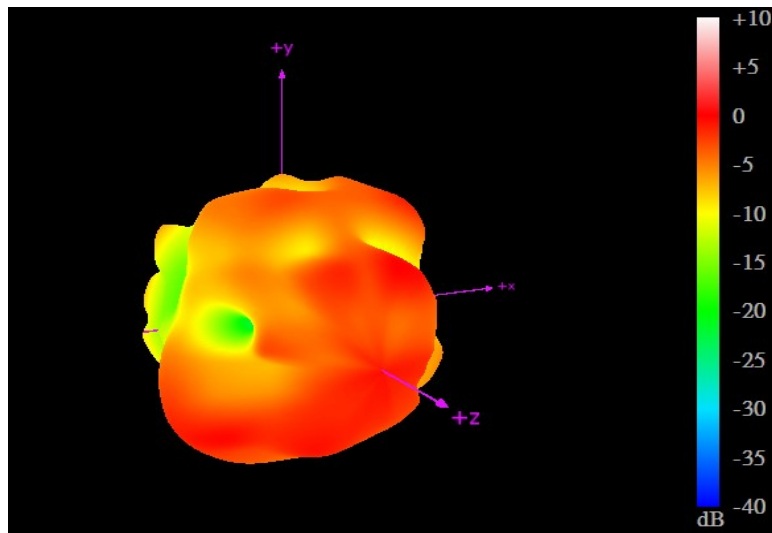
5550MHz
