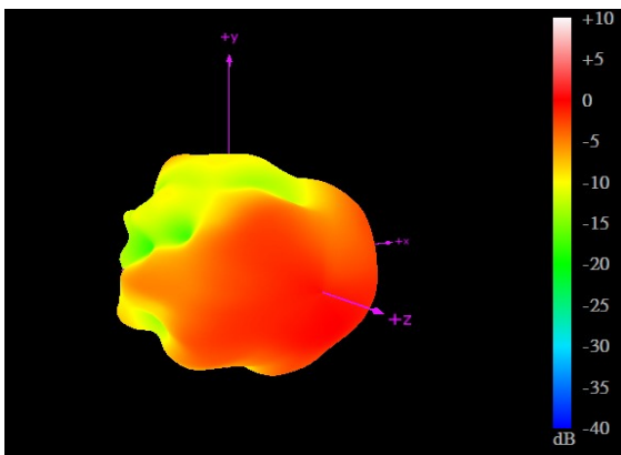
1710MHz
