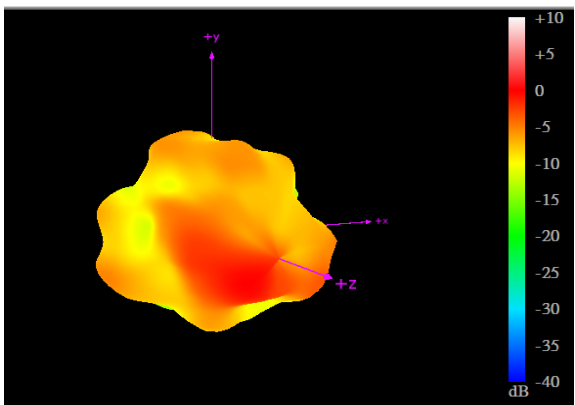
2690MHz
