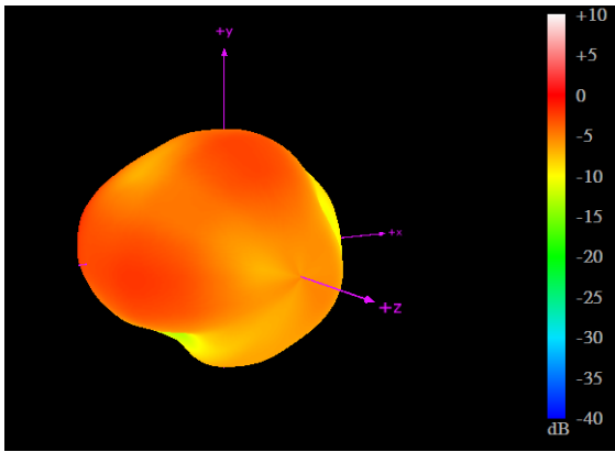
704MHz
