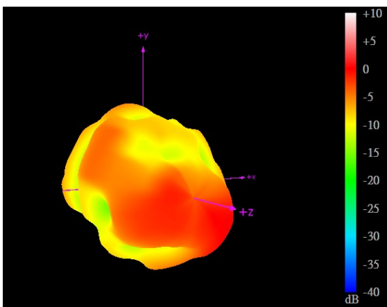
2690MHz
