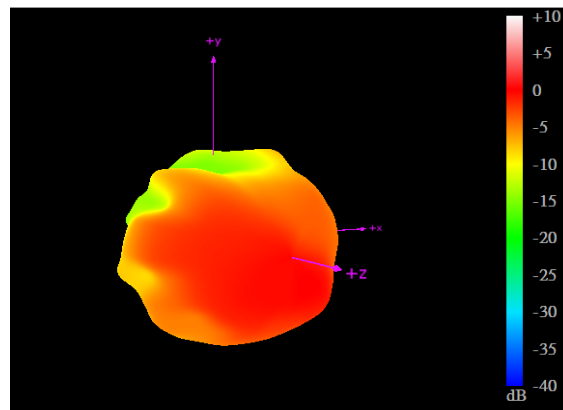
2170MHz
