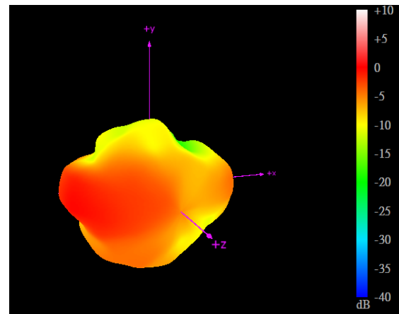
2170MHz
