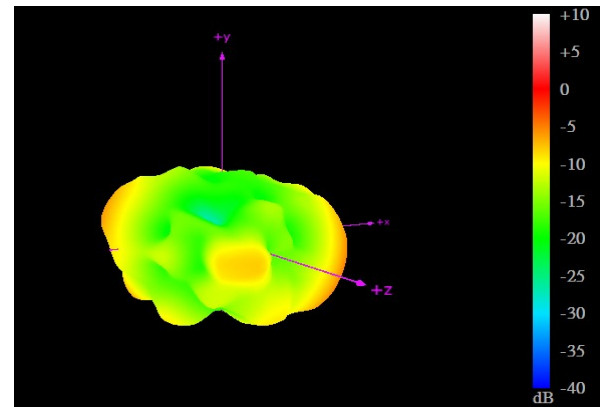
2170MHz
