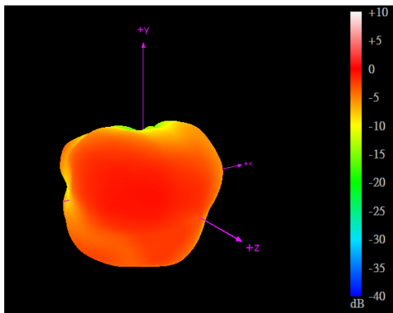
1710MHz
