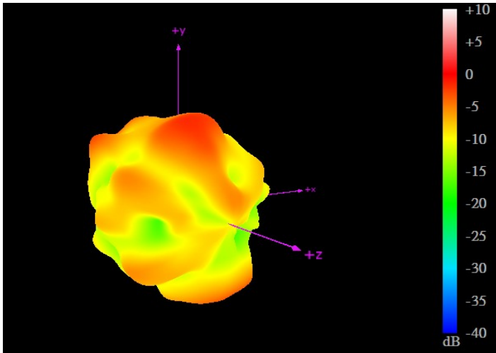
2450MHz
