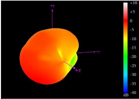
704MHz
