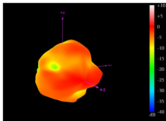
3500MHz
