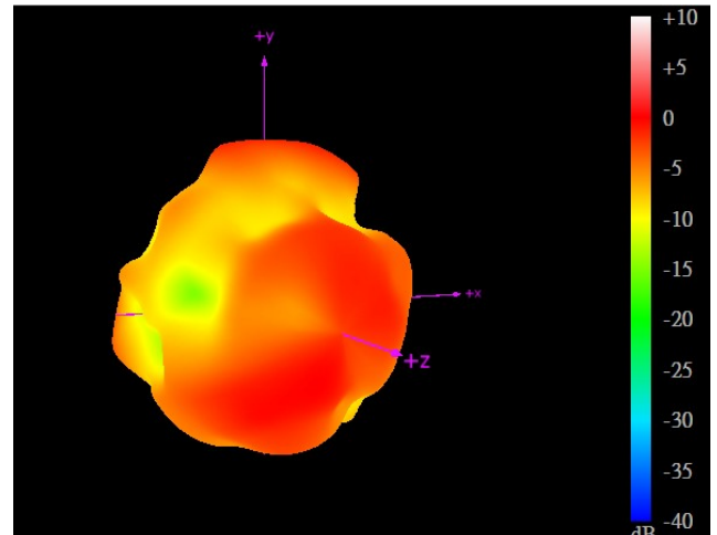
5550MHz
