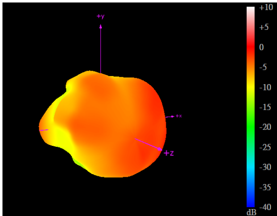
1710MHz
