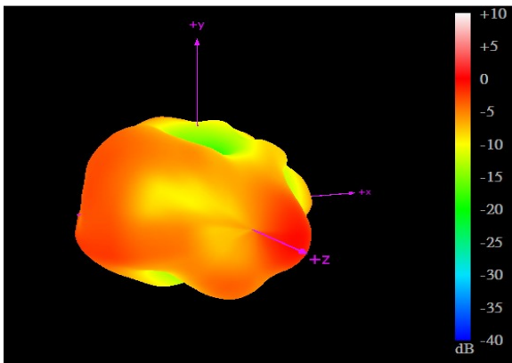
1710MHz
