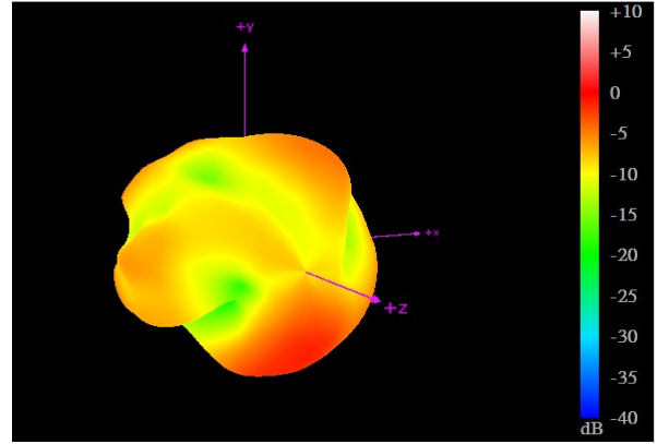
960MHz
