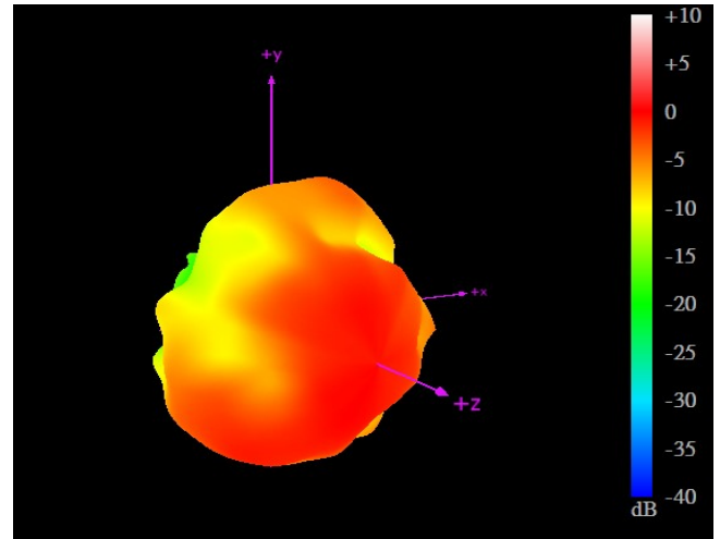
5550MHz
