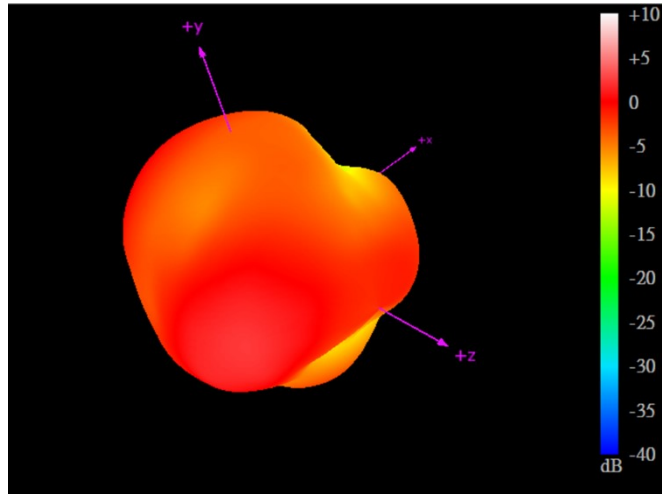
1561MHz
