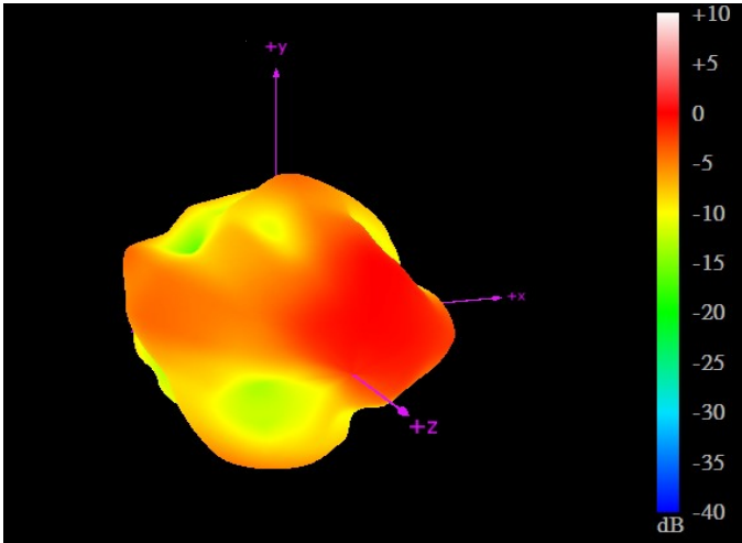
2450MHz
