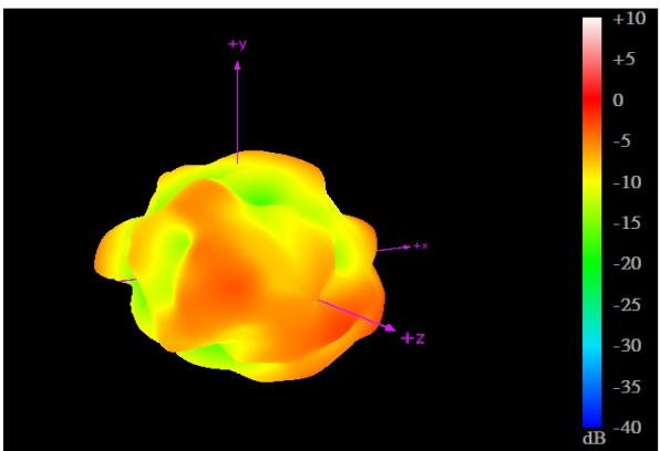
2690MHz
